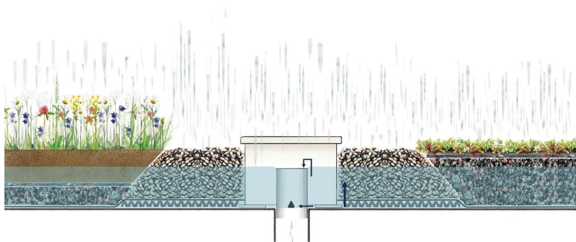
Figur 8. Illustrasjonen er hentet fra www.bergknapp.no og viser oppbygningen av et blågrønt tak med restriktor i midten, semi-intensivt tak med engvegetasjon til venstre og ekstensivt tak med sedummatter lengst til høyre.
