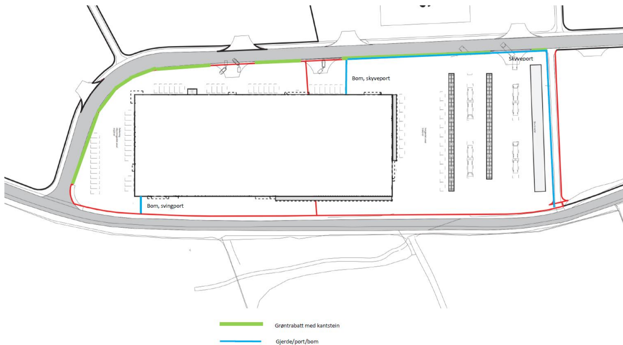
Figur 2. Utomhus-skisse for nytt byggevarehus på Raglamyr.
